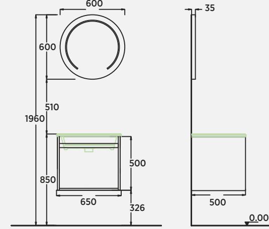
Capitol 65 cm Lavabo Dolabı Washbasin Cabinet | Mobile Lavabo Capitol 60 cm Aydınlatmalı Fonksiyonlu Ayna Illuminated Mirror With Function Specchio Con Funzioni Illuminato
