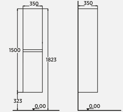
Capitol 35 cm Boy Dolabı Tall Cabinet | Armadio Alto
