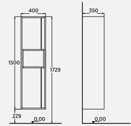
Allure 40 cm Boy Dolabı Tall Cabinet | Armadio Alto
