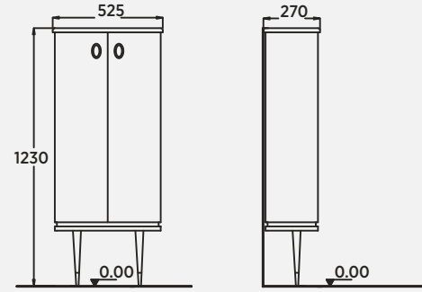
Blanc 50 cm Boy Dolabı Tall Cabinet | Armadio Alto
