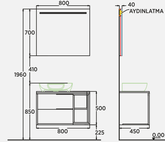
Allure 80 cm Lavabo Dolabı Washbasin Cabinet | Mobile Lavabo Ortak 80 cm Aydınlatmalı Ayna Illuminated Mirror | Specchio Illuminato
