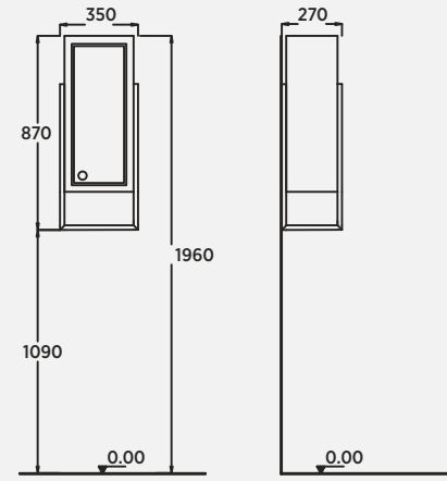
Loft 35 cm Üst Yan Dolap Top Side Cabinet | Armadietto Laterale Superiore
