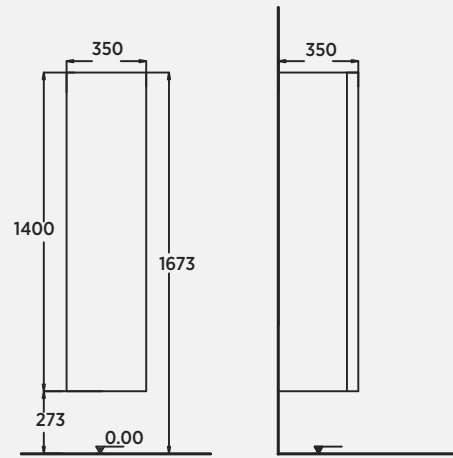
Drexel 35 cm Boy Dolabi | Tall Cabinet | Armadio Alto
