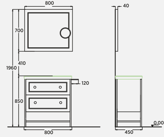
Loft 80 cm Lavabo Dolabi Washbasin Cabinet | Mobile Lavabo Loft 80 cm Fonksiyonlu Aydınlatmalı Ayna Illuminated Mirror With Function Specchio Con Funzioni Illuminato
