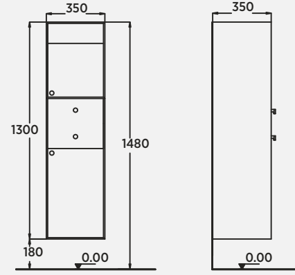
Liv 35 cm Boy Dolabı Tall Cabinet | Armadio Alto
