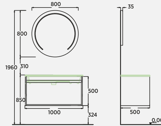
Capitol 100 cm Lavabo Dolabı Washbasin Cabinet | Mobile Lavabo Capitol 100 cm Aydınlatmalı Fonksiyonlu Ayna Illuminated Mirror With Function Specchio Con Funzioni Illuminato
