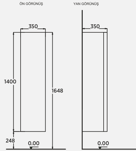
Bold 35 cm Boy Dolabı Tall Cabinet | Armadio Alto
